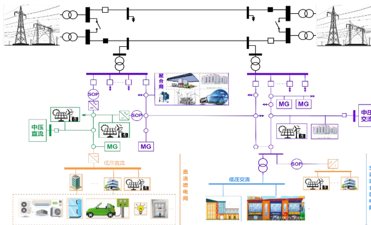
图 12 分布式智能电网
